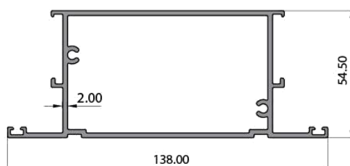
VF3304 Ngang cánh (đổ chân) cửa đi mở quay 2.033 Kg/m
