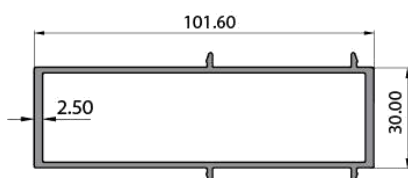
VF3304 Ngang cánh (đổ chân) cửa đi mở quay 2.033 Kg/m
