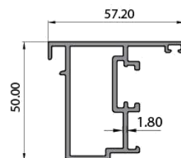
VF3323 Đổ động cửa đi 1.053 Kg/m
