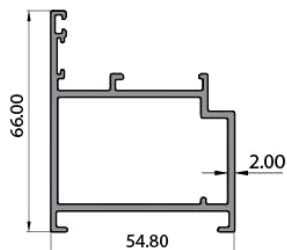
VF3328 Khung bao cửa đi mở quay 1.225 Kg/m
