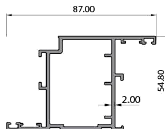
VF3332 Cánh cửa đi mở trong 1.442 Kg/m
