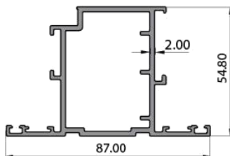
VF3303 Cánh cửa đi mở ngoài 1.441 Kg/m
