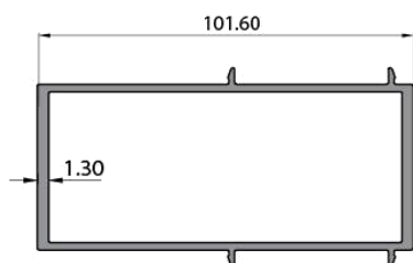
VF3310 Nối thẳng tăng cứng 1.313 Kg/m
